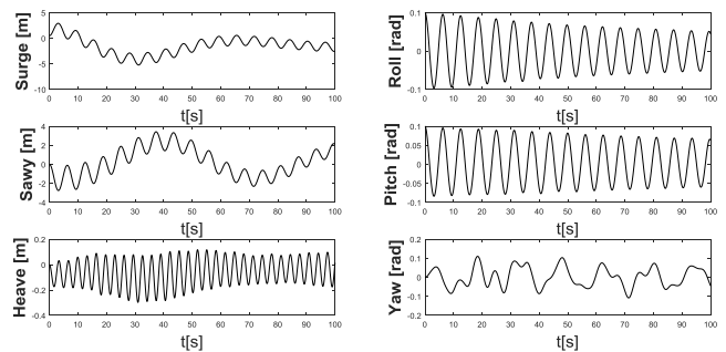
شکل ۴- ارتعاشات آزاد توربین بادی شناور با پایه TLP
