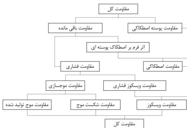
شکل ۳- انواع مقاومت در شناورها [۱۰].
