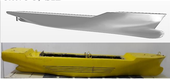
شکل ۴- مدل شناور KCS
