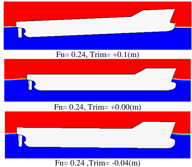
شکل ۱۱- نمایش تریم‌های مختلف
