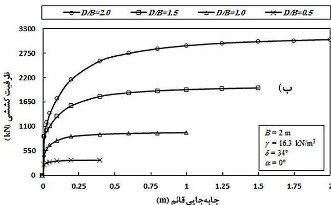
شکل ۶- منحنی‌های بار-جابه‌جایی مدل‌های پی لبه‌دار؛ الف) نتایج مدل‌سازی فیزیکی، ب) نتایج مدل‌سازی عددی
