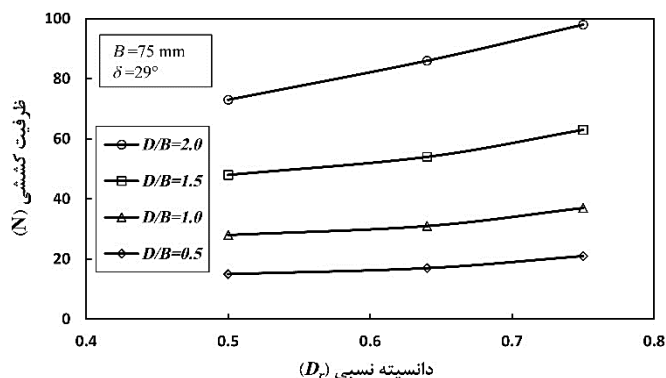
شکل ۹- تاثیر دانسیته نسبی ماسه بر میزان ظرفیت کششی پی
