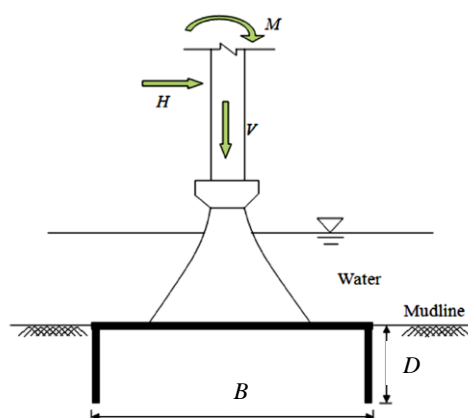
شکل ۱- نمایی از کاربرد پی‌های لبه‌دار تحت انواع بارگذاری [۱]
