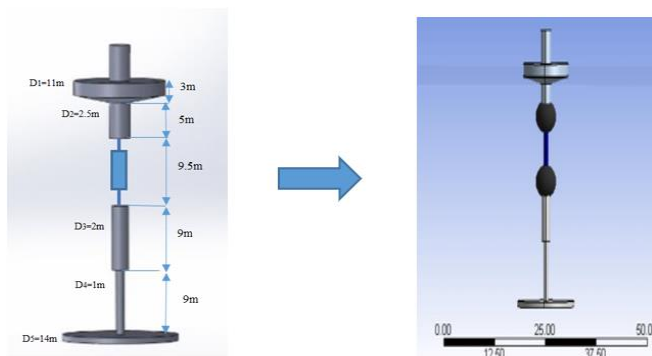
شکل ۶ - نحوه مدل سازی مبدل جاذب دو بدنه‌ای در نرم‌افزار انسیس آکوا
