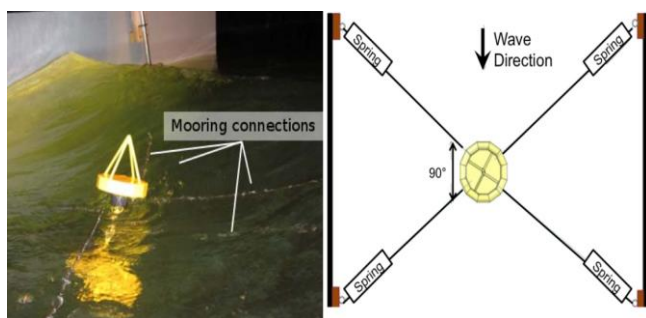
شکل ۵- مهار مبدل جاذب نقطه ای دوبدنه ای در استخر موج دانشگاه سن دیگو [۱۹]
