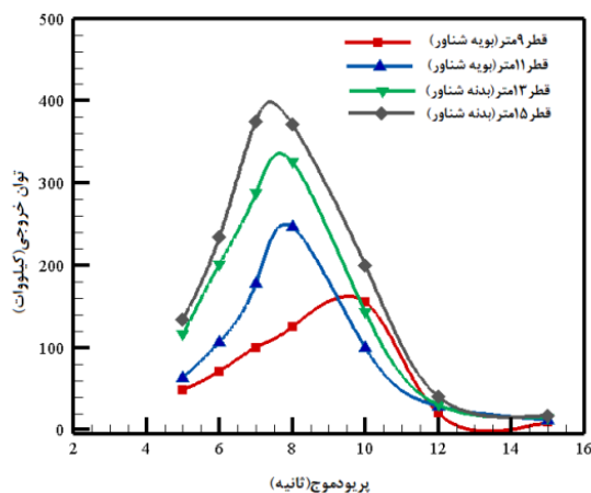
شکل ۱۴- تاثیر تغییرات قطر بدنه شناور بر میزان توان
