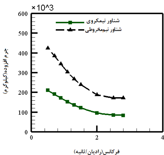
شکل ۱۳- ب): نمودار ضریب میرایی هیدرودینامیکی - فرکانس موج برخوردی برای دو شکل نیم‌کروی و نیم مخروطی
