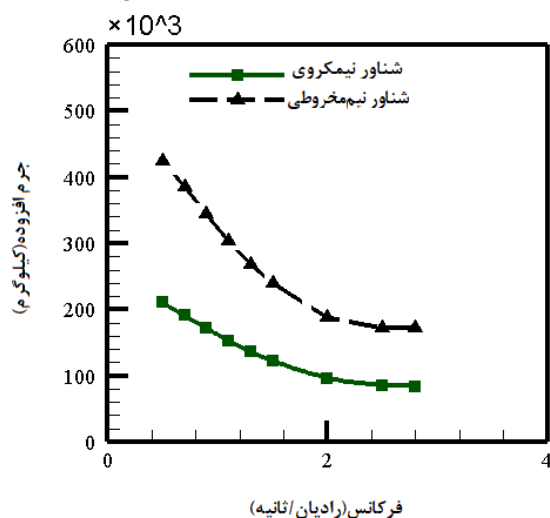
شکل ۱۳- الف): نمودار جرم افزوده - فرکانس موج برخوردی برای دو شکل نیم‌کروی و نیم مخروطی
