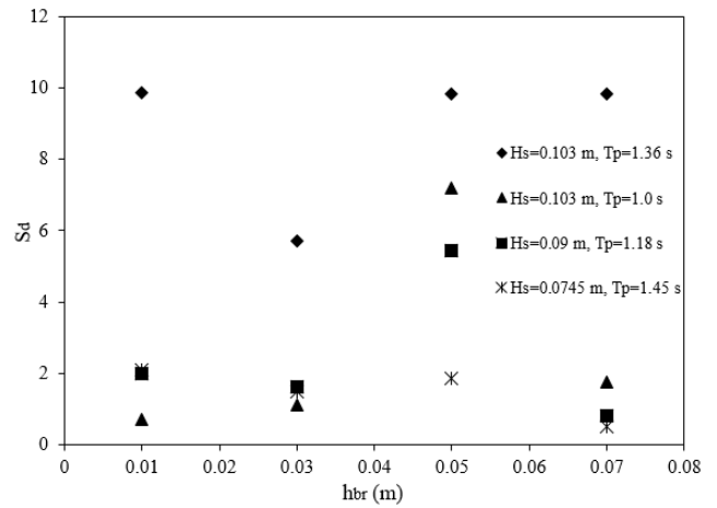
شکل ۶- تأثیر تراز سکو از سطح ایستایی بر روی پارامتر آسیب موج-شکن سکویی چندلایه برای ترکیب‌های متفاوت امواج
