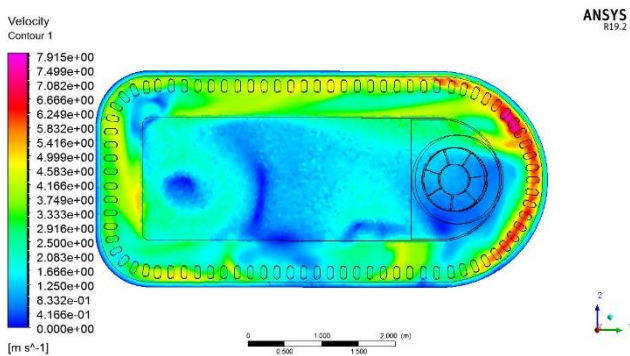
شکل ۱۵- کانتور توزیع سرعت برای قطعه با شیب صفر درجه
