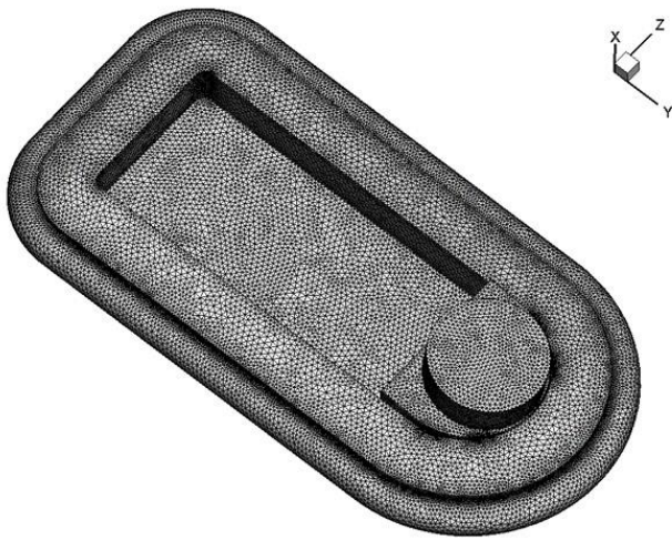
شکل ۸- مش بدنه هاورکرافت
