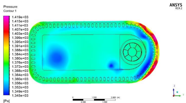
شکل ۱۱- کانتور توزیع فشار در یک صفحه افقی در نزدیکی سطح زیر هاورکرافت اولیه
