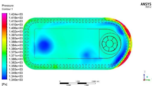
شکل ۱۴- کانتور توزیع فشار برای قطعه با شیب صفر درجه
