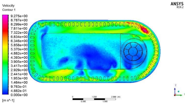
شکل ۱۹- کانتور توزیع سرعت برای قطعه با شیب ۶ درجه
