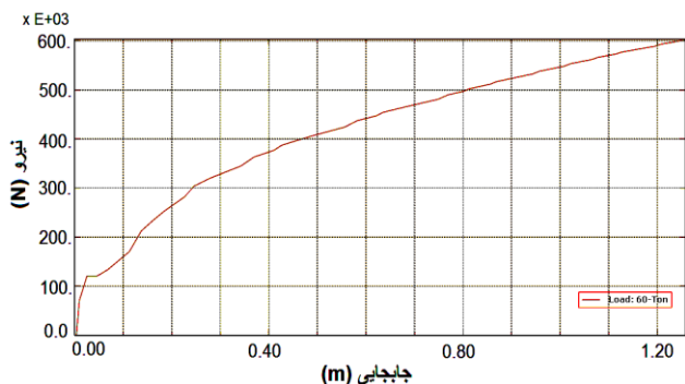
شکل ۲۵-نمودار نیرو - جابجایی در اثر اعمال نیروی ۶۰ تن
