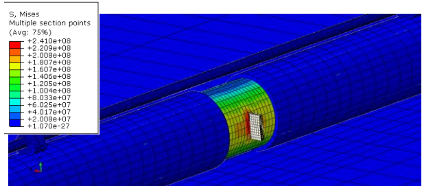
شکل ۱۷- تنش وارده به خط لوله در اثر اعمال نیروی ۳۰ تنی
