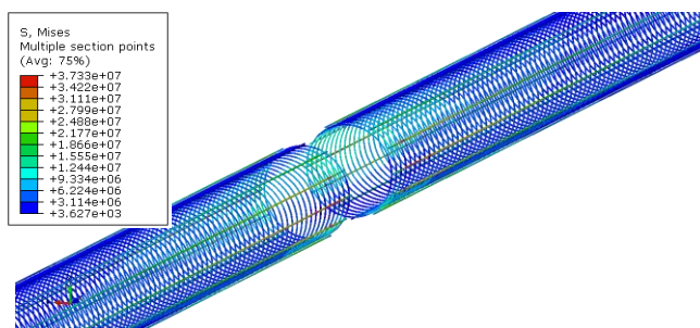
شکل ۱۴- تنش وارده به میلگردها در اثر اعمال نیروی ۱۰ تنی
