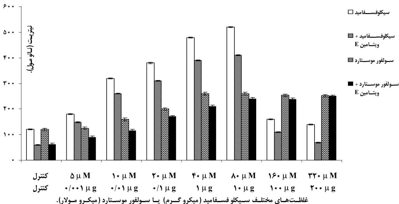
شکل ۱: مقایسه مقدار نیتریک اکساید مترشحه توسط ماکروفاژهای صفاقی موش در پاسخ به غلظت‌های مختلف سیکلوفسفامید، سولفور موستارد در حضور یا عدم حضور ویتامین E.
