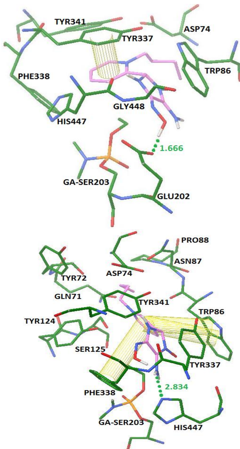
شکل-۴. برهمکنش های ۱۰ (بالا) و ۱۱ (پایین) با ساختار کریستالی AChE مهار شده با تابون با کد 2JF0. برهمکنش های \pi-\pi و هیدروژنی نمایش داده شده است
