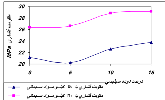
شکل ۲. منحنی تغییرات مقاومت فشاری ۷ روزه بر حسب درصد دوده سیلیس
