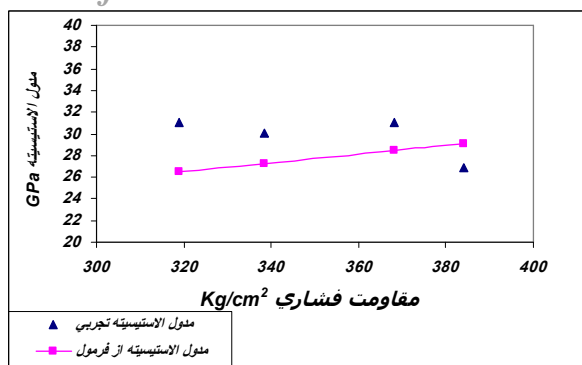
شکل ۴. محاسبه مدول الاستیسیته بر حسب مقاومت فشاری از فرمول دوم و مقایسه با نتایج نمونه ها
