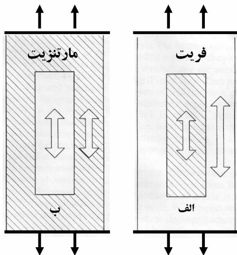
شکل ۶. طرحی شماتیک از ساختار دوفازی تحت تغییر شکل.
