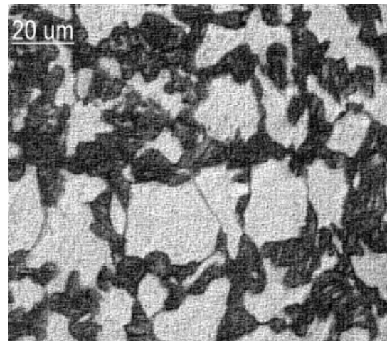
شکل ۲. ریزساختار حاصل از آنیل میان بحرانی به مدت ۱۲۰ ثانیه در دمای ۷۹۰ °C، که حاوی ۴۸٪ مارتنزیت سیاه رنگ می‌باشد.
