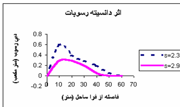
شکل ۶. اثر دانسیته رسوبات در انتقال رسوب موازی ساحل
