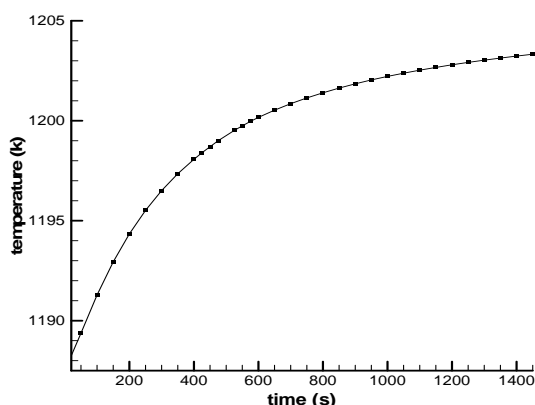
شکل ۱۴. تغییرات زمانی دما در الکترولیت در موقعیت حدود
