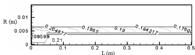
شکل ۱۵. کانتورهای کسر جرمی اکسیژن در پیل سوختی
