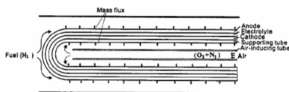
شکل ۱. نمای دوبعدی از اجزاء و نحوه عملکرد تک سلول پیل
