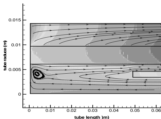
شکل ۱۲. خطوط جریان در کانال های سوخت و هوا در انتهای
