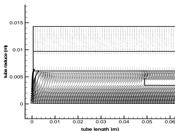
شکل ۱۱. بردارهای سرعت در کانال های سوخت و هوا در
