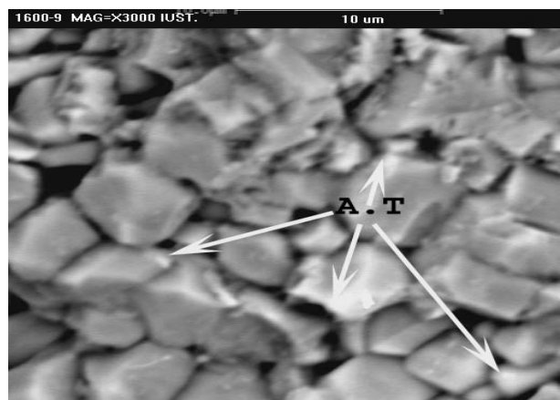
شکل ۱۰. تصویر ریزساختاری نمونه حاوی ۹ درصد TiO 2 پخته شده در دمای (۱۶۰۰ °C/۲h) در بزرگنمایی (x۳۰۰۰)
