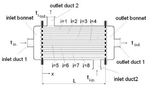
شکل ۱. مبدل حرارتی پوسته و لوله [۱۲]
