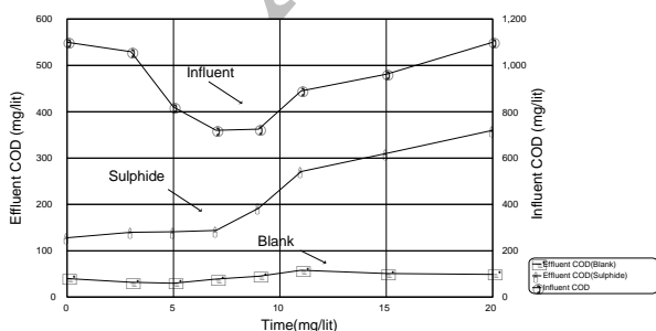
شکل ۵. تغییرات COD بر حسب زمان در غلظت ۱۰۰ ppm
