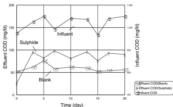
شکل ۳. تغییرات COD بر حسب زمان در غلظت ۳۰ ppm
