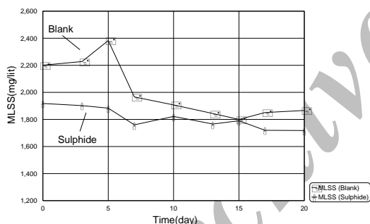
شکل ۴. تغییرات MLSS بر حسب زمان در غلظت ۳۰ ppm
