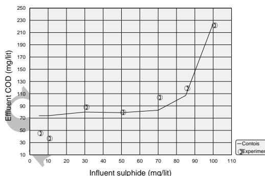
شکل ۹. مقایسه COD خروجی مدل کن تویس با نتایج تجربی سیستم حاوی سولفید
