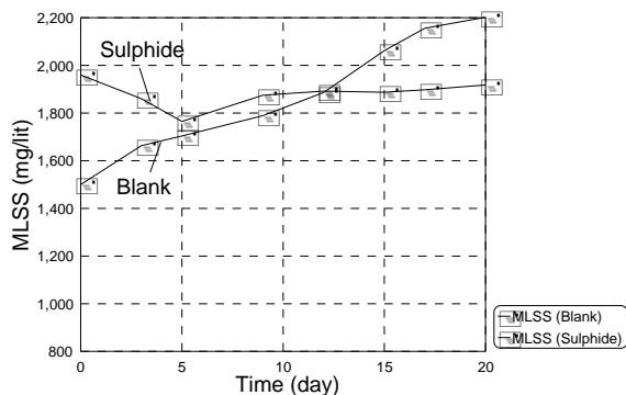
شکل ۲. تغییرات MLSS بر حسب زمان در غلظت ۱۰ ppm
