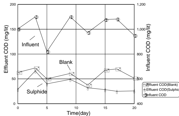
شکل ۱. تغییرات COD بر حسب زمان در غلظت ۱۰ ppm
