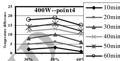
شکل ۱۹. اختلاف دما برحسب نسبت پرشدن برای زمان های مختلف در توان ۴۰۰ وات و نقطه ۴ توسط شبیه سازی فرآیند
