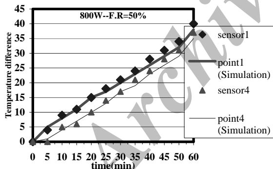
شکل ۲۳. اختلاف دما برحسب زمان برای نقطه شماره ۴ در توان ۸۰۰ وات و نسبت پرشدن ۵۰٪ در دو حالت تجربی و شبیه سازی
