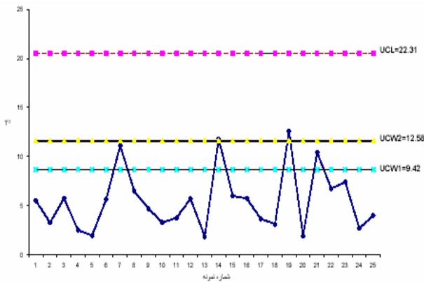
شكل ۲. نمودار كنترل برای داده‌های اولیه
