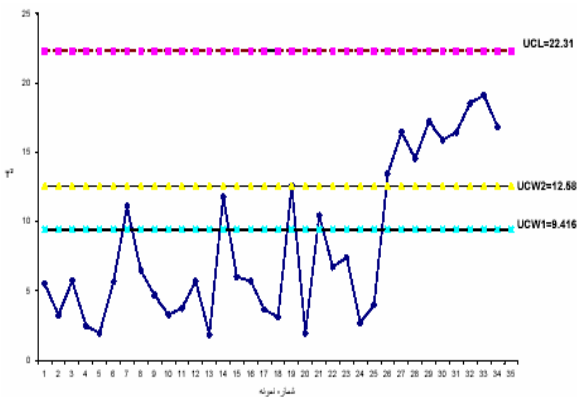
شكل ۳. نمودار كنترل پس از تغییر در میانگین مشخصه‌های
