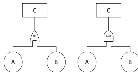
شکل ۵. درخت خرابی مربوط به گره های A,B,C با
