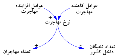
شکل ۵- تفکیک عوامل اثرگذار بر روی نرخ مهاجرت به عوامل افزایشده و کاهشده مهاجرت
