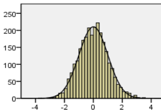
نمودار ۱. هیستوگرام توزیع نرمال
