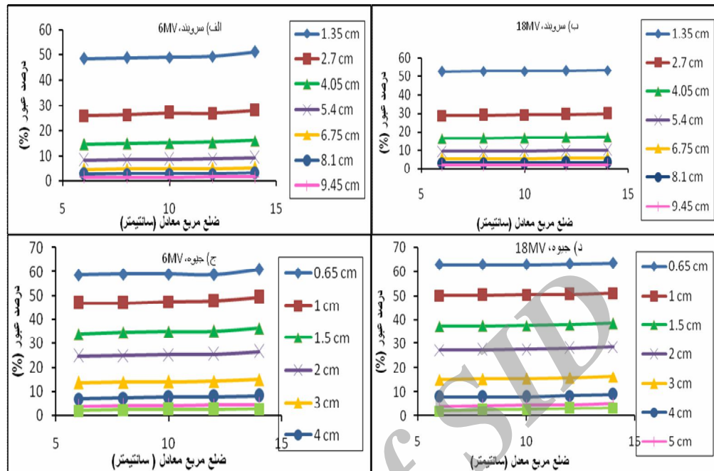
شکل 7. مقادیر فاکتور عبور برحسب ضلع میدان درمانی برای ضخامت‌های مختلف سروبنده: الف) انرژی 6MV، ب) انرژی 18MV و جیوه: ج) انرژی 6MV، د) انرژی 16MV
