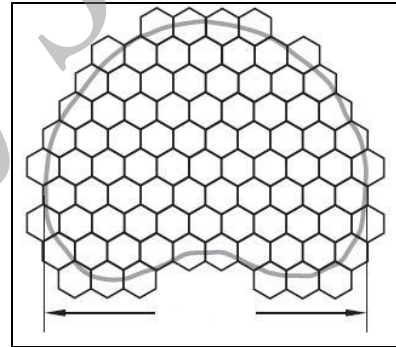
شکل 3. تطابق کانتور درمانی با قطر d با چینش لوله‌های جیوه (سطح مقطع شش ضلعی)
