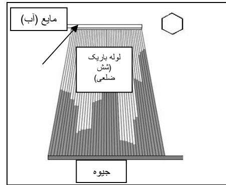
شکل 6. طرح شماتیک سیستم تعدیل کننده جیوه‌ای طراحی شده
