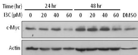
شکل ۳. نتایج یکی از ۳ مرتبه آزمون وسترن بلات برای بررسی اثر I3C در غلظت‌های مشخص بر بیان پروتئین c-Myc پس از ۲۴ و ۴۸ ساعت مجاورت با سلول‌های NALM-6
