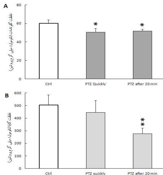
نمودار ۲. اثر تشنج پتیلن تترازول بر تغییرات گلوتامات و گابای هیپوکامپی.
