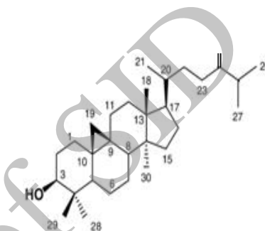
ترکیب ۱: سیکلوآرتان-۲۴-متیلین-۳-ا ۱
