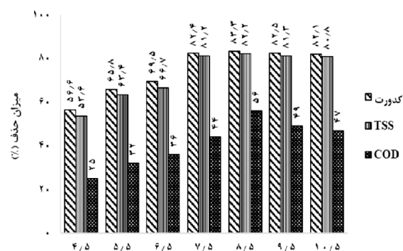
نمودار ۲- تأثیر مقادیر مختلف pH بر راندمان حذف کدورت، TSS و COD توسط پلی‌آلومینیوم کلراید به عنوان منعقدکننده (غلظت ثابت برای منعقدکننده = ۴۰۰ میلی‌گرم بر لیتر)
