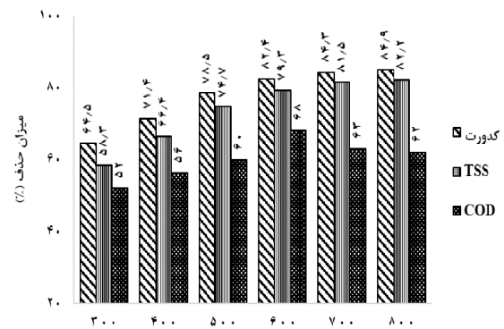
نمودار ۳- تأثیر غلظت های مختلف سولفات آلومینیوم بر راندمان حذف کدورت، TSS و COD در pH بهینه برابر ۸/۵
