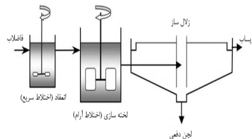
شکل ۱- شماتیک فرآیند انعقاد شیمیایی [۱۸]
