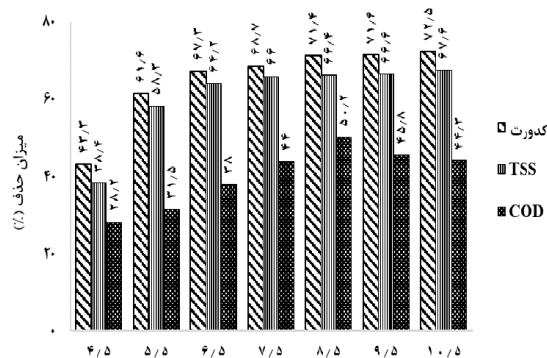
نمودار ۱- تأثیر مقادیر مختلف pH بر راندمان حذف کدورت، TSS و COD توسط سولفات آلومینیوم به عنوان منعقدکننده غلظت ثابت برای منعقدکننده = ۴۰۰ میلی‌گرم بر لیتر
