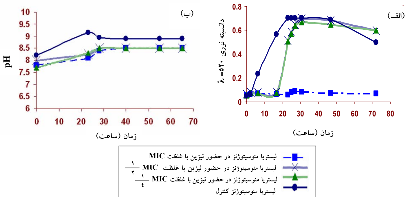
شکل ۳ منحنی رشد لیستریا منوسیتوژنز در حضور نیزین با غلظت های MIC، MIC و MIC (الف) و تغییرات pH محیط کشت در حضور غلظت های MIC، MIC و نیزین (ب)
