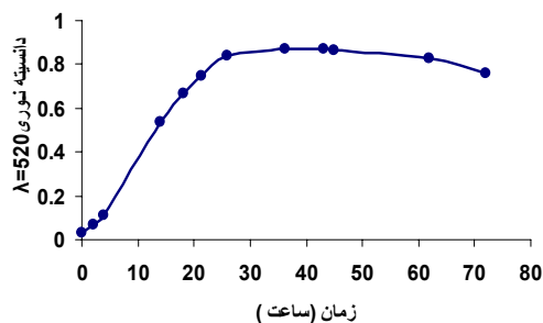
شکل ۱ منحنی رشد باکتری لیستریا منوسیوتوزنز جدا شده از شیر بدون حضور ماده نگهدارنده
