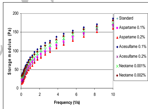
شکل ۷ تأثیر شیرین کننده‌های سنتزی بر روی مدول ذخیره یا G' محلولهای گوار ۱/۵٪
