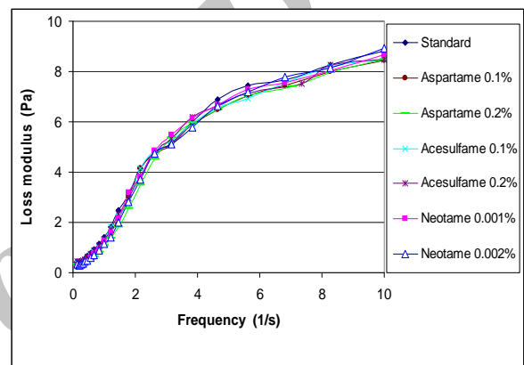
شکل ۲ تأثیر شیرین کننده های سنتزی بر روی مدول افت G'' محلولهای گوار ۰/۵٪
