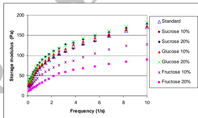
شکل ۷ تأثیر شیرین‌کننده‌های طبیعی بر روی مدول ذخیره یا G' محلولهای گوار ۱/۵٪
