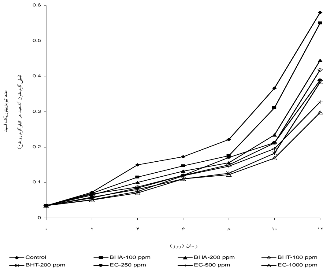
شکل ۵ روند تغییرات میزان عدد تیوباربتوریک اسید تیمارهای مختلف حاوی عصاره‌ی اتانولی میوه‌ی بلوط، آنتی اکسیدان‌های سنتزی و نمونه‌ی شاهد طی نگهداری در دمای ۷۰°C.
