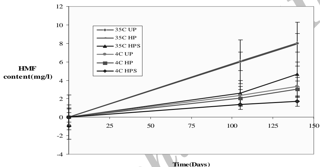
شکل ۸ میزان تجمع هیدروکسی متیل فورفورال در طی دوره نگهداری در دو دمای ۳۵°C و (۴±۲)°C.
