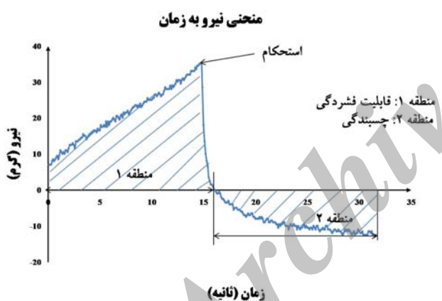
شکل ۱ منحنی تیبیک نیرو به زمان جهت تعیین ویژگی‌های بافت نمونه‌های پخشینه با نسبت‌های مختلف ژلاتین ماهی به پکتین.
