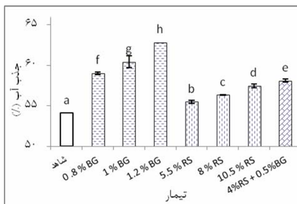
شکل ۱ رابطه جایگزینی سطوح مختلف بتاگلوکان و نشاسته مقاوم با جذب آب خمیر
