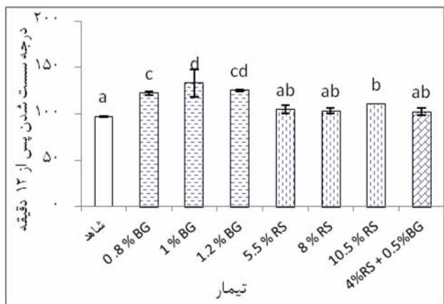
شکل ۴ رابطه جایگزینی سطوح مختلف بتاگلوکان و نشاسته مقاوم با درجه سستی شدن خمیر
