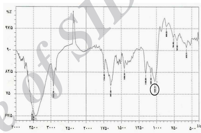
شکل ۴ نمودار FTIR مربوط به نان پوشش داده شده با آلزینات سدیم پس از سه روز نگهداری
