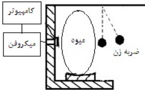
شکل ۱ سامانه صوتی
