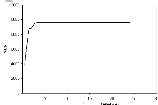
شکل ۵. ارتباط بین درجه متورم شدن و زمان غوطه وری برای هیدروژل اتصال عرضی شده PAA همراه با همزدن نمونه در ۲۵ °C.
