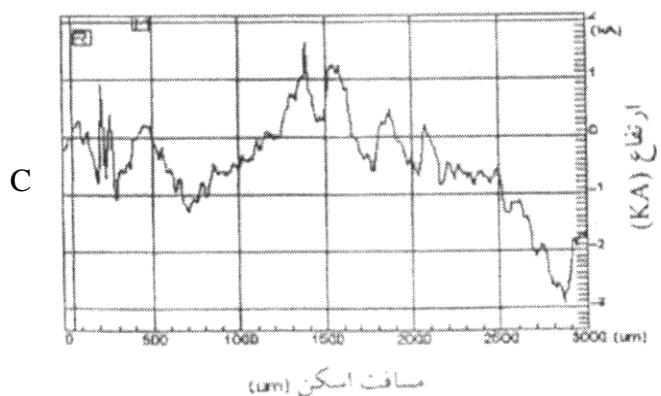
تصویر ۲: اسکن های تهیه شده توسط دستگاه پروفیلومتر از سیم های ارتودنسی فولاد زنگ نزن. A- امریکن ارتودنتیکس B- ارتوتکنولوژی C- آلستار
