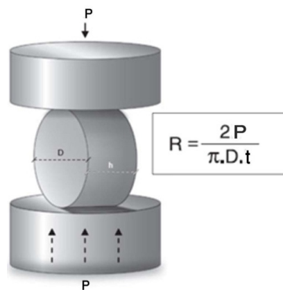
تصویر ۲: نمایی از تست استحکام کششی قطری
