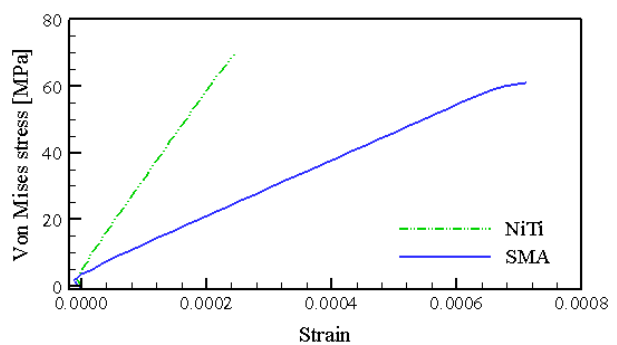
نمودار ۱: تغییرات تنش در مقابل کرنش در دو نوع ایمپلنت
