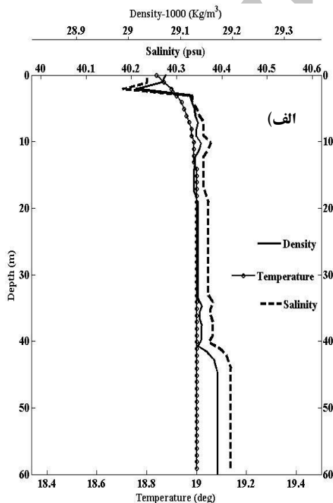
شکل ۳. الف) شرایط اولیه توزیع قائم کمیت‌های فیزیکی آب خلیج فارس ب) شرایط اولیه و شرایط مرز باز توزیع قائم کمیت‌های فیزیکی آب در دریای عربی.
