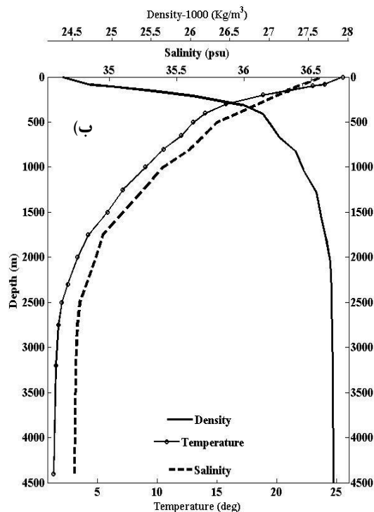
شکل ۳. الف) شرایط اولیه توزیع قائم کمیت‌های فیزیکی آب خلیج فارس ب) شرایط اولیه و شرایط مرز باز توزیع قائم کمیت‌های فیزیکی آب در دریای عربی.
