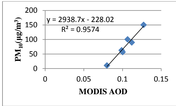
نمودار ۱. همبستگی میان عمق اپتیکی حاصل از سنجنده MODIS ماهواره ترا و داده‌های ایستگاه‌های محیط‌زیست برای تابستان 2008-2013
