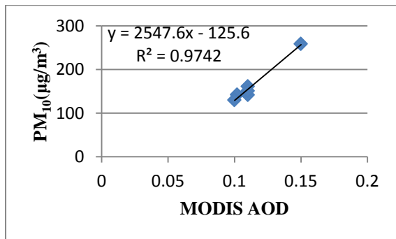
نمودار ۲. همبستگی میان عمق اپتیکی حاصل از سنجنده MODIS ماهواره آکوا و داده‌های ایستگاه‌های محیط‌زیست برای تابستان 2008-2013
