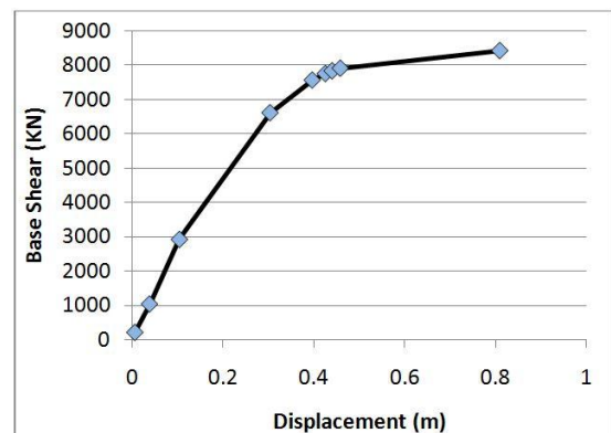
شکل ۶. منحنی ظرفیت موج افزایشی برای راستای ۱۸۰ درجه
