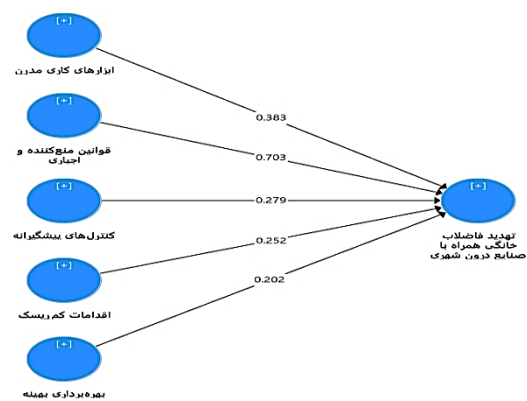
شکل (۴): آزمون مدل تهدید فاضلاب خانگی و راهکارهای مرتبط با آن در حالت ضرایب استاندارد
