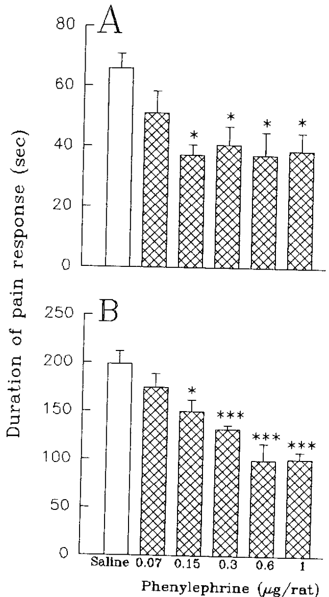
شکل ۵- اثر بی‌دردی وابسته به دوز فنیل افرین در آزمایش فرمالین - سالیین (۳ μg/rat, ICV) و یا فنیل افرین (۰/۰۷، ۰/۱۵، ۰/۳، ۰/۶، ۱/۵، ۱/۰ μg/rat, ICV) ۵ دقیقه قبل از آزمایش فرمالین به صورت ICV تزریق گردید. اثر بی‌دردی طی ۰ تا ۵ دقیقه (شکل A فاز حاد) و ۶۰-۱۵ دقیقه (شکل B فاز مزمن) پس از تزریق فرمالین ثبت گردید. هر نقطه میانگین ± SEM، ۷ آزمایش می‌باشد. * P < ۰/۰۵ و *** P < ۰/۰۰۱ اختلاف از گروه سالیین مربوطه را نشان می‌دهد.
