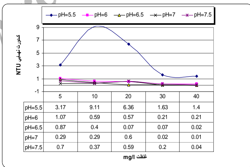
نمودار شماره ۵- کدورت نهایی در غلظت ها و pH های مختلف منعقدکننده پلی آلومینیوم کلراید با کدورت اولیه ۸۰ NTU
