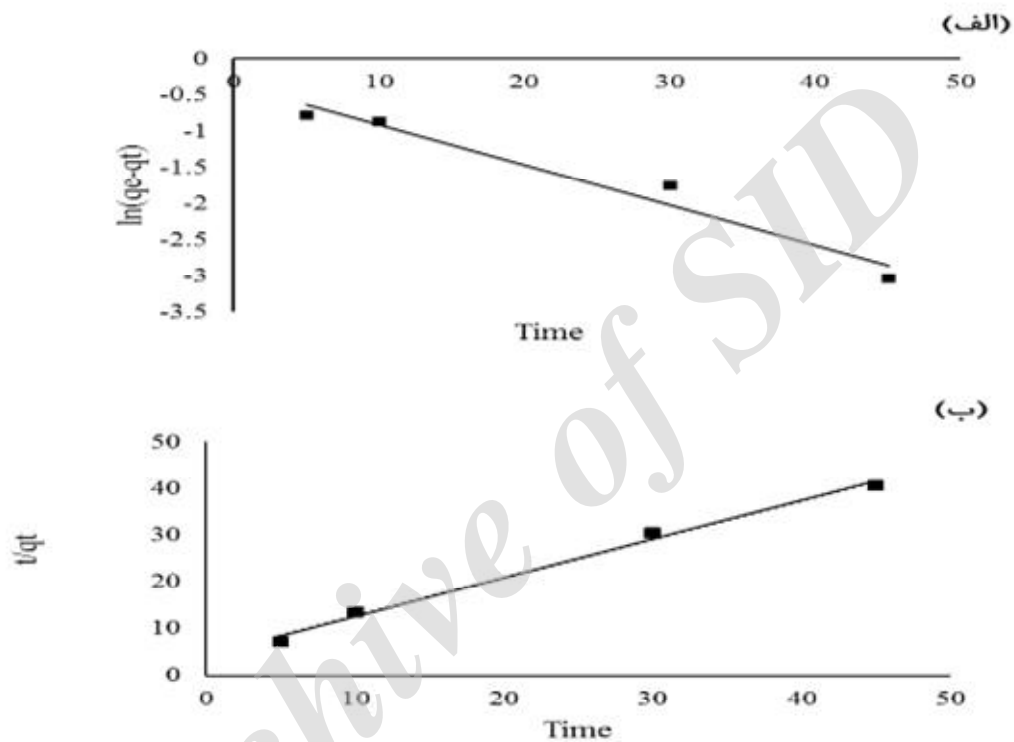
شکل ۱۱: نمودار شبه سینتیک درجه اول (الف) شبه سینتیک درجه دوم (ب) برای جذب کلرپیریفوس روی کیتوزان گرافن اکساید
