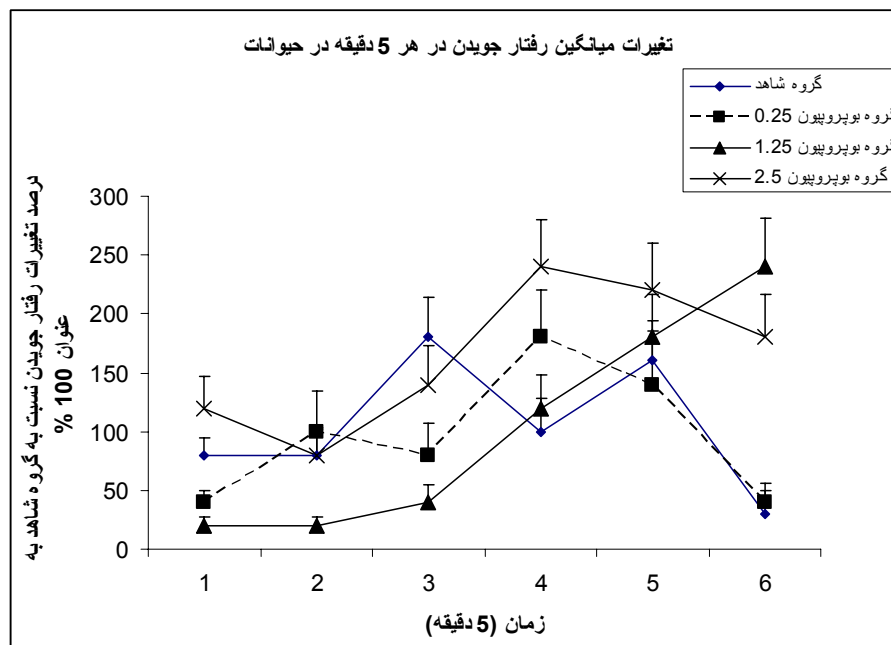
شکل شماره (۴): نمودار میانگین تغییرات در رفتار جویدن در گروه‌های مختلف موش‌های تحت آزمایش در بازه‌های زمانی ۵ دقیقه‌ای. در این نمودار میانگین رخدادهای رفتار جویدن در کل زمان گروه شاهد به عنوان صد در صد انتخاب شده و تغییرات رفتار نسبت به آن مقایسه شده است.
