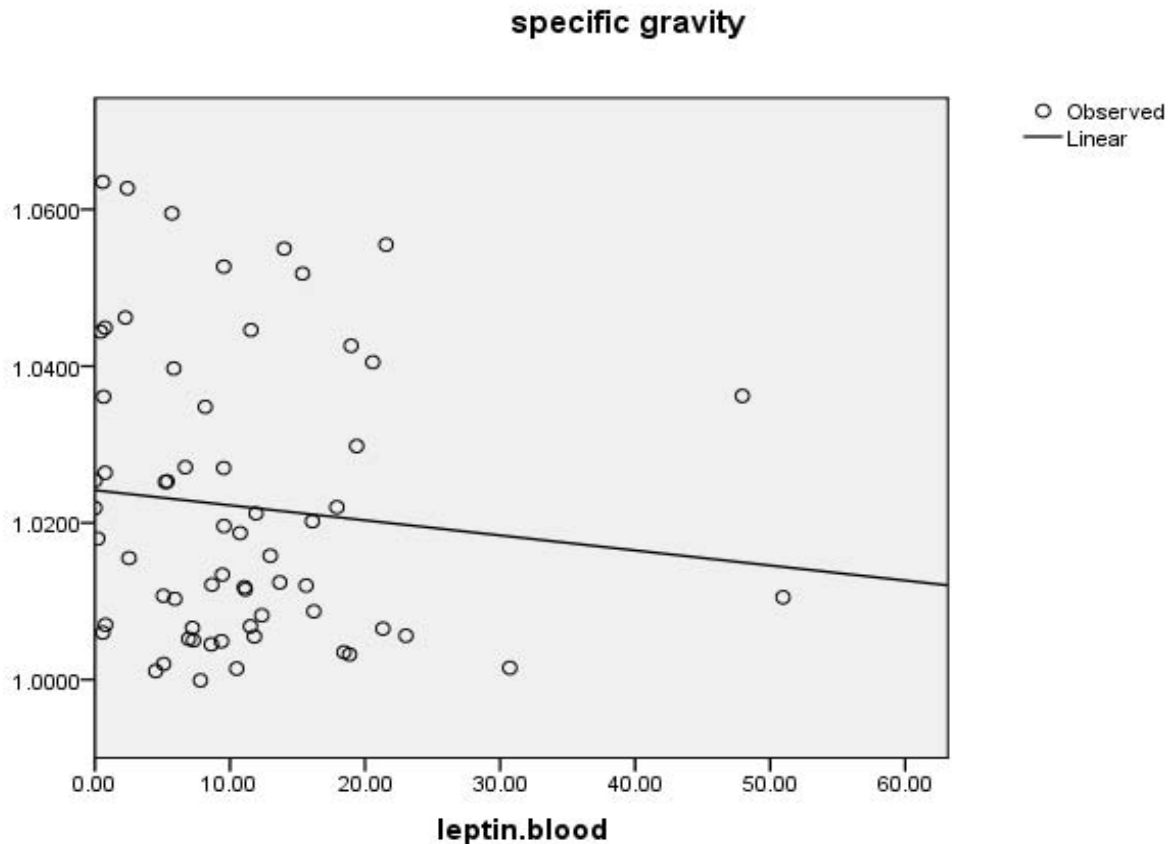
شکل شماره (۳): تاثیر سطح لپتین خون مادر بر وزن حجمی شیر
