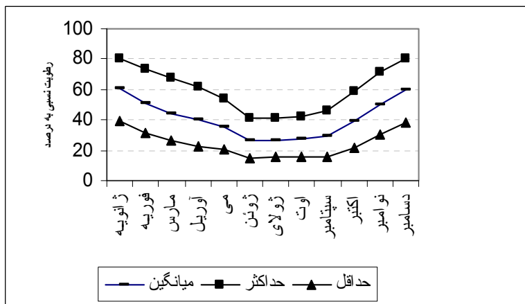
نمودار ۳: حداقل، میانگین و حداکثر رطوبت نسبی ایستگاه اصفهان مأخذ: سازمان هواشناسی کل کشور
