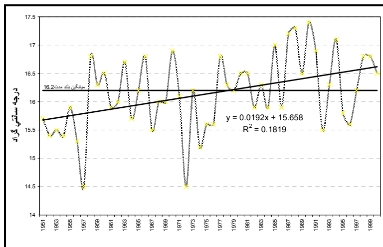
نمودار ۲: رژیم سالانه دما و میانگین بلندمدت و سری زمانی دمای اصفهان (۱۹۵۱-۲۰۰۰) مأخذ داده‌ها: سازمان هواشناسی کل کشور
