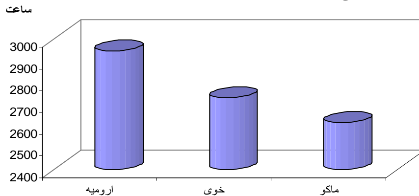
نمودار ۲: میانگین ساعات آفتابی سالانه در ایستگاههای مورد مطالعه (۱۹۸۹-۲۰۰۳) *ایستگاههای سلماس، کهریز، قوشچی، مرز سرو و میرآباد فاقد آمار ساعات آفتابی می باشند.
