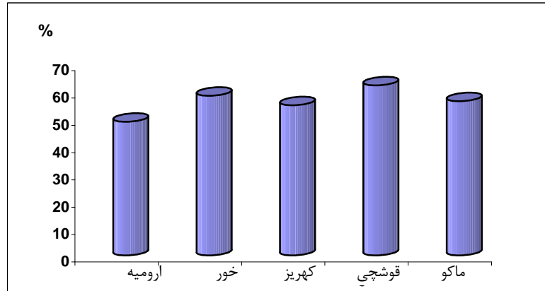
نمودار ۱: میانگین رطوبت نسبی سالانه در ایستگاههای مورد مطالعه (۱۹۸۹-۲۰۰۳) *ایستگاههای سلماس و مرز سرو و میرآباد فاقد آمار رطوبت نسبی می باشند.
