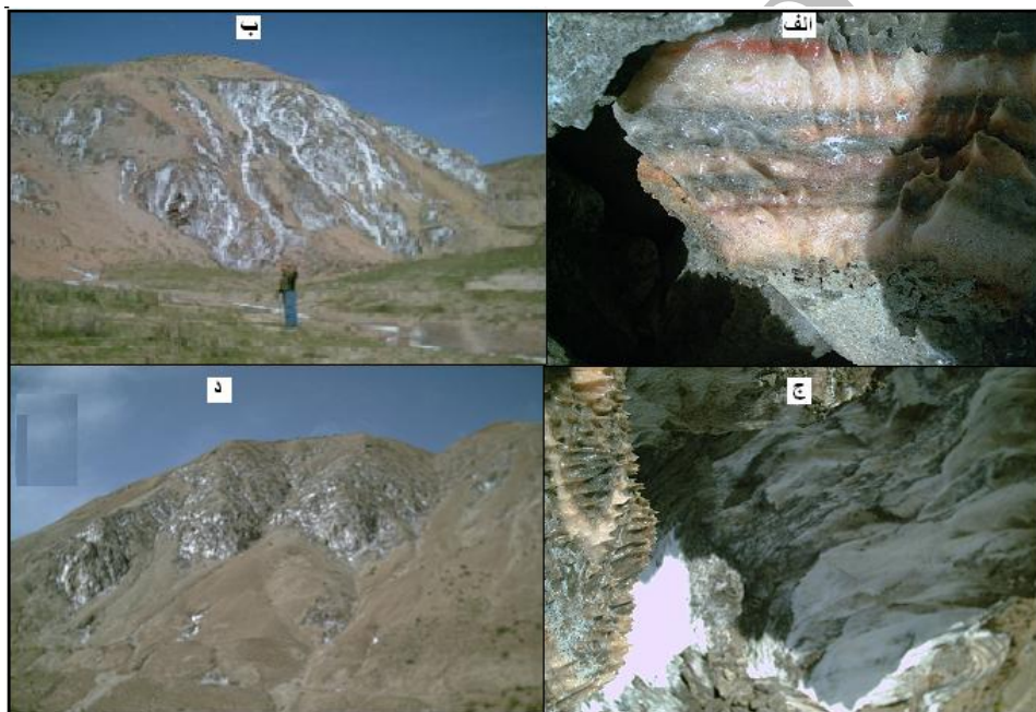
شکل ۷: تصویری از لایه‌های رنگی نمک (الف) - گنبد ایوند (ب) سینک حول و شیارهای انحلالی (ج) - گنبد منور (د)
